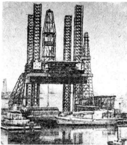
Плавающая буровая платформа для бурения на шельфе
