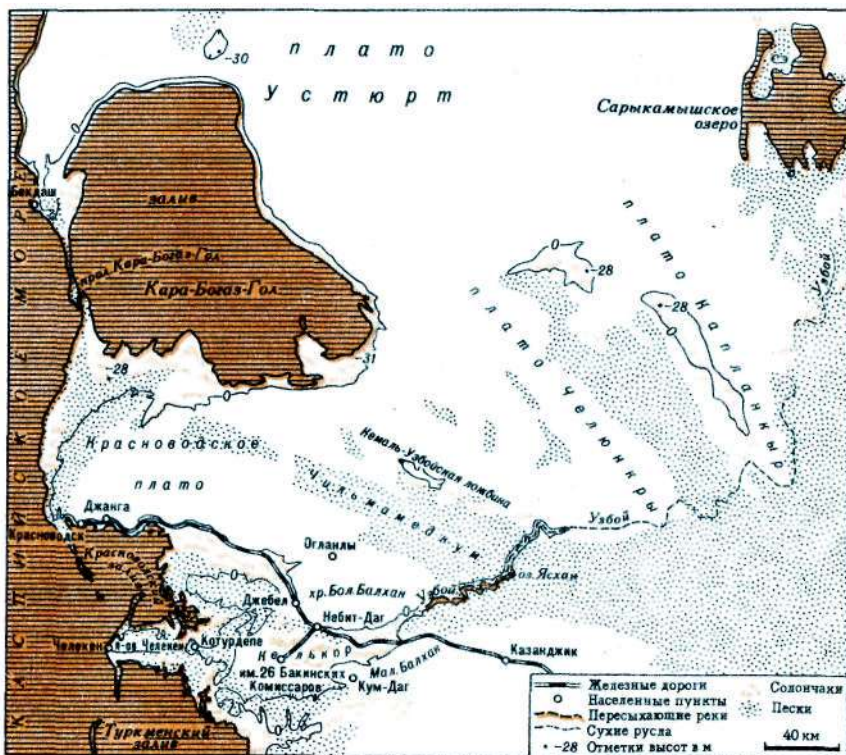
Русло Узбоя
