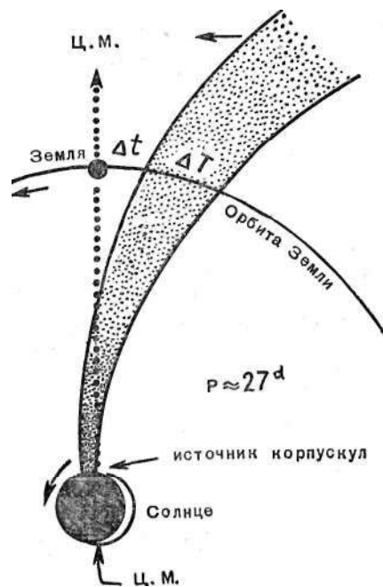
Схема периодического попадания Земли в поток корпускул, идущий от активной области на поверхности Солнца (по Э. Р. Мустелю)
