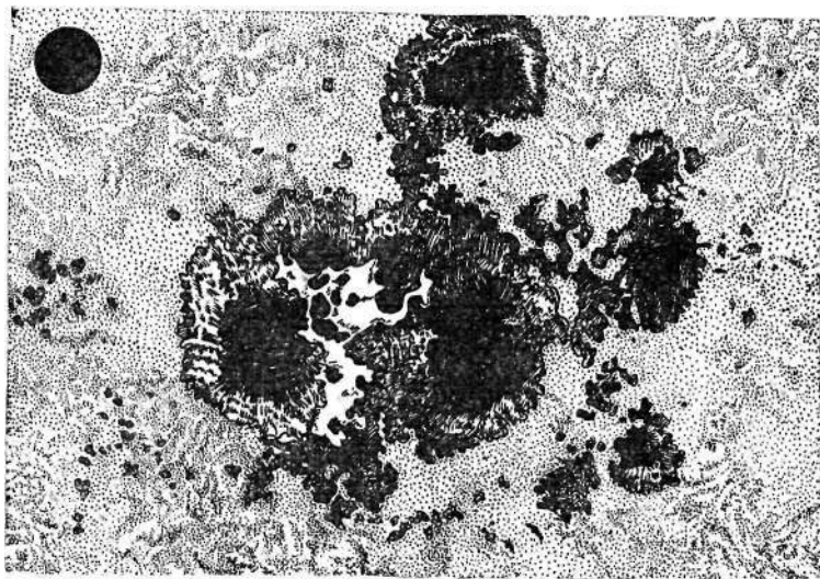
Группа солнечных пятен, наблюдавшаяся 6 августа 1917 г. в обсерватории на горе Вильсон. (Черный диск в левом углу показывает сравнительные размеры Земли)
