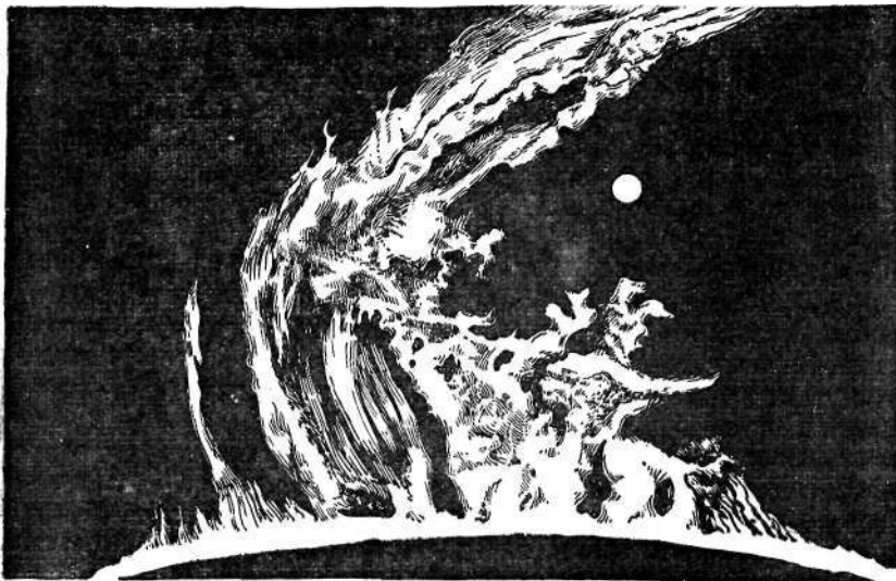
Солнечный протуберанец высотой 235 000 километров. Сфотографирован 9 июля 1917 г. в обсерватории на горе Вильсон. (Белый кружок — сравнительные размеры Земли)
