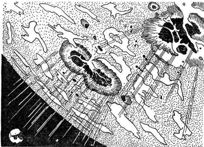
Схема корпускулярных излучений солнечных пятен (внизу слева относительные размеры Земли)
